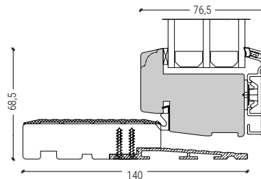
Underkarm og ramme til smalrammet terrassedør
