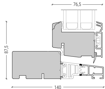
Bundkarm og ramme
