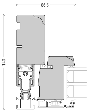
Venstre sidekarm og ramme
