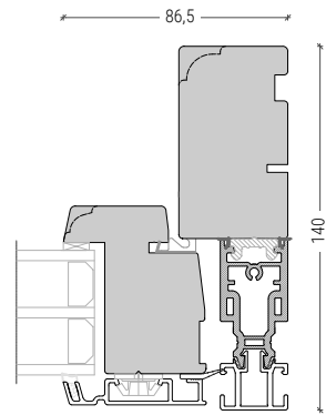
Højre sidekarm og ramme
